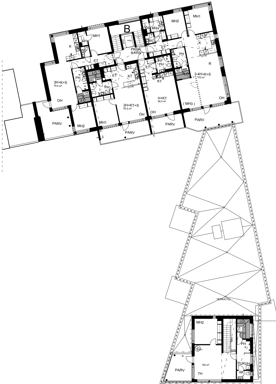
Pohjapiirros n. 1:250 6. kerros
