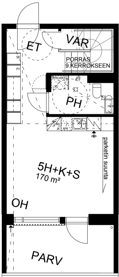
pohjapiirros 8.krs n. 1:100
