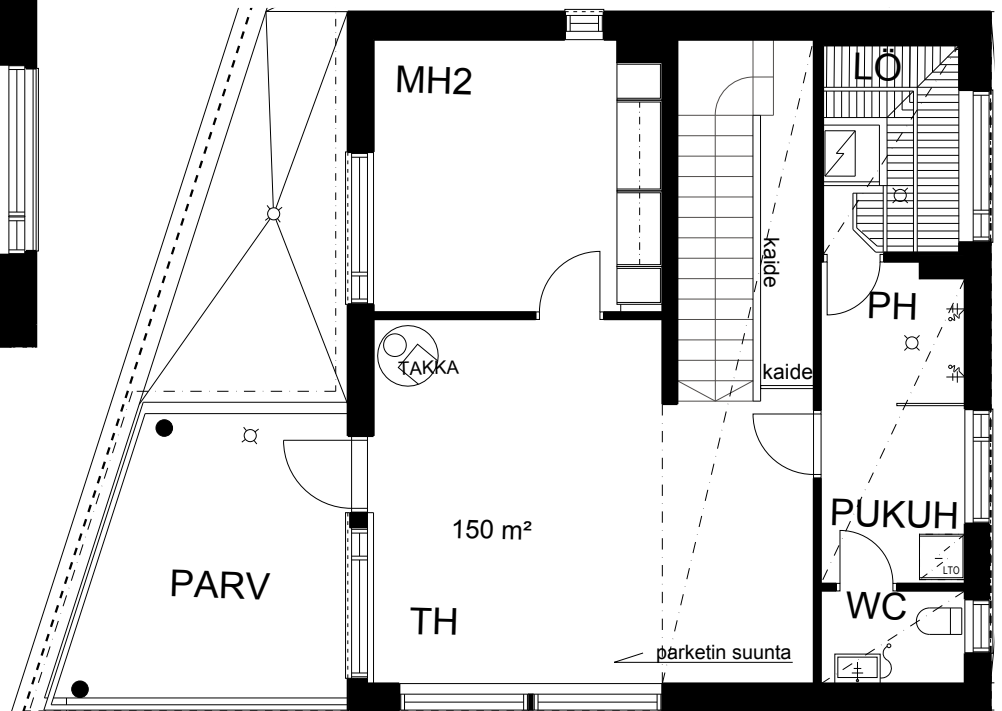
pohjapiirros 6.krs n. 1:100
