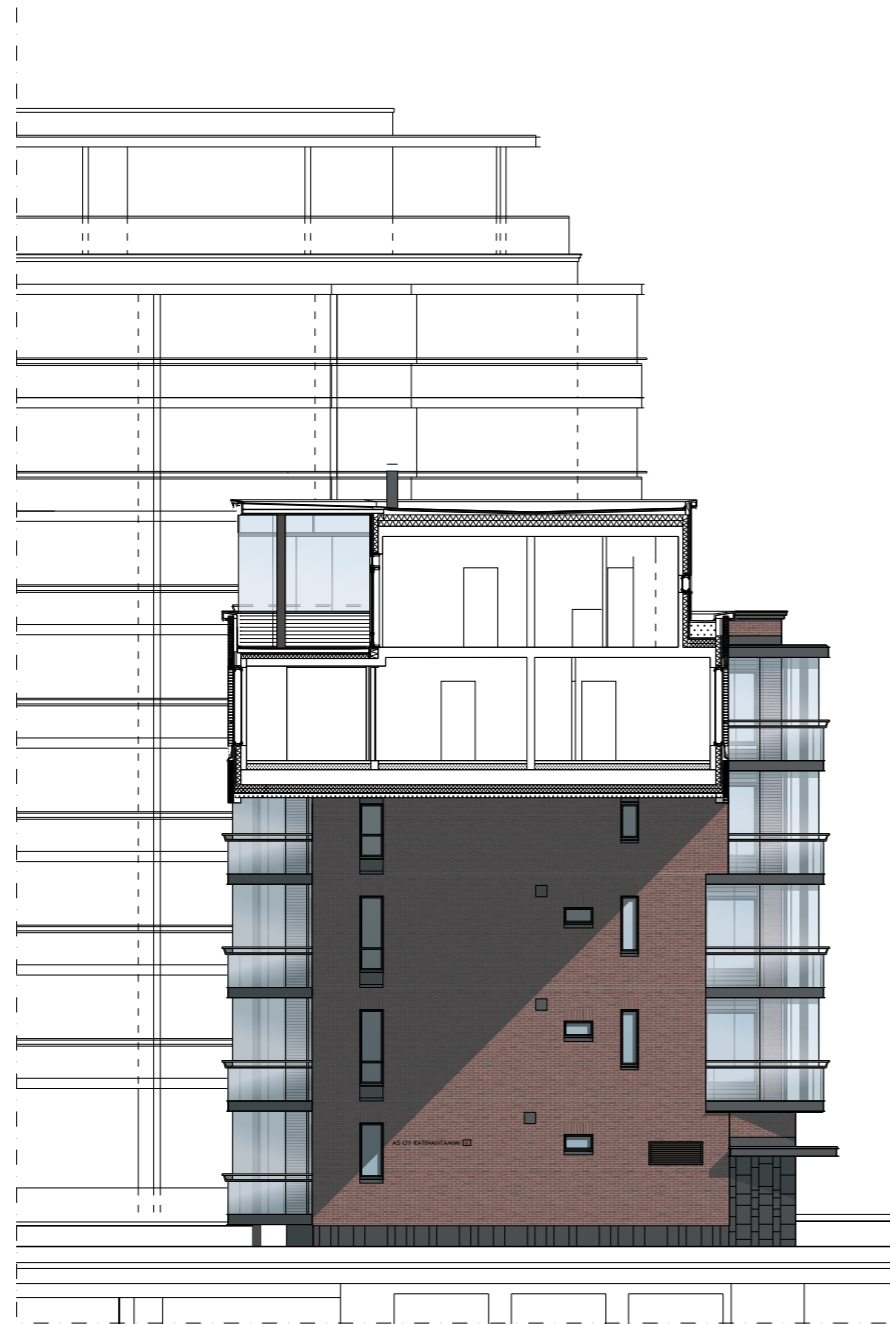
JULKISIVU ETELÄÄN AS OY RATINANTAMMI
