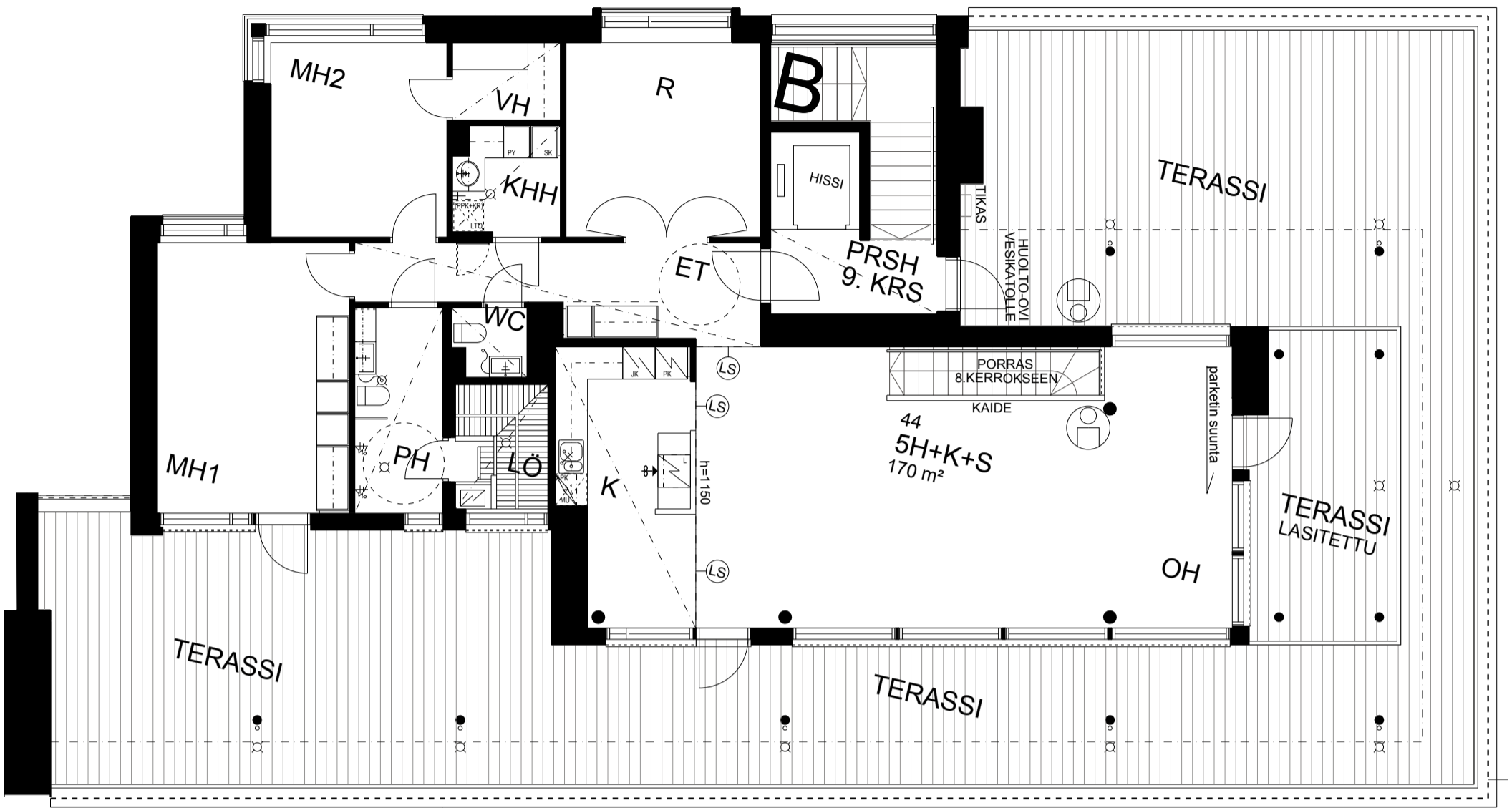
pohjapiirros 9.krs n. 1:100
